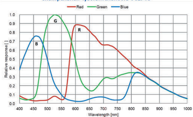
Спектральная чувствительность VC174C
