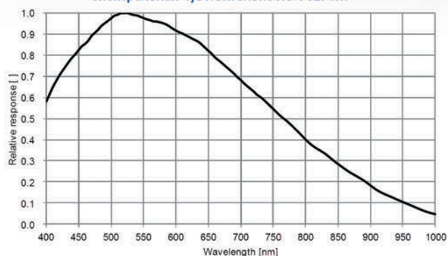
Спектральная чувствительность VC174C
